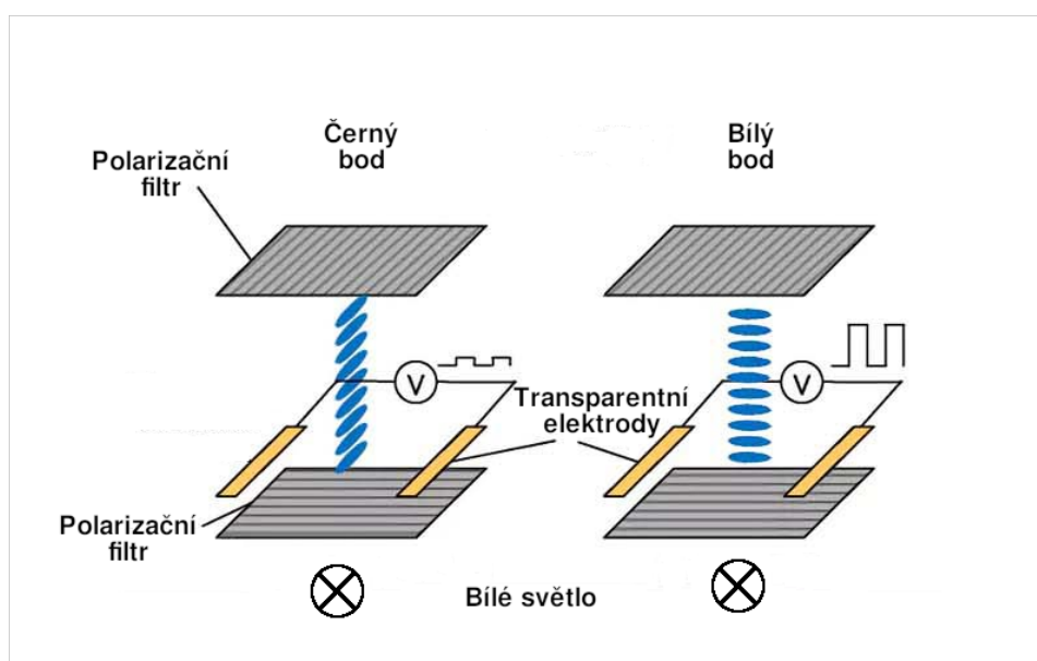
Obrázek 4: Princip činnosti IPS displeje
