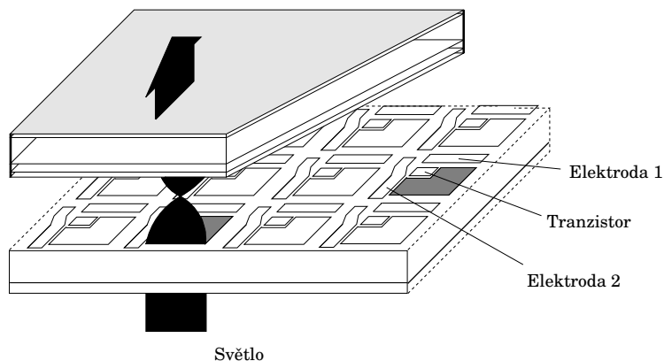
Obrázek 7: Struktura TFT displeje
