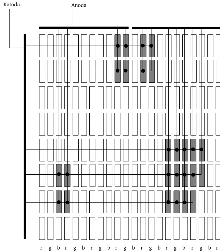
Obrázek 6: Struktura pasivního displeje
