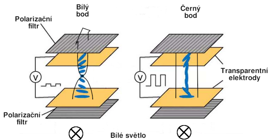
Obrázek 3: Princip činnosti TN displeje
