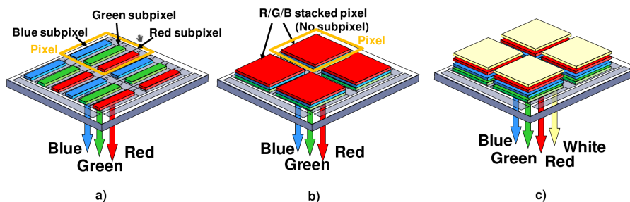
Obrázek 11: RGB OLED
