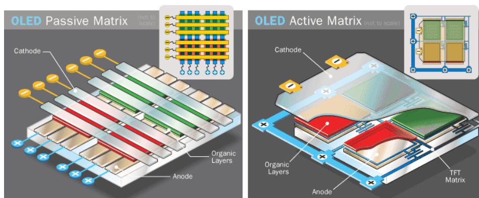
Obrázek 12: Rozdíl mezi PMOLED a AMOLED
