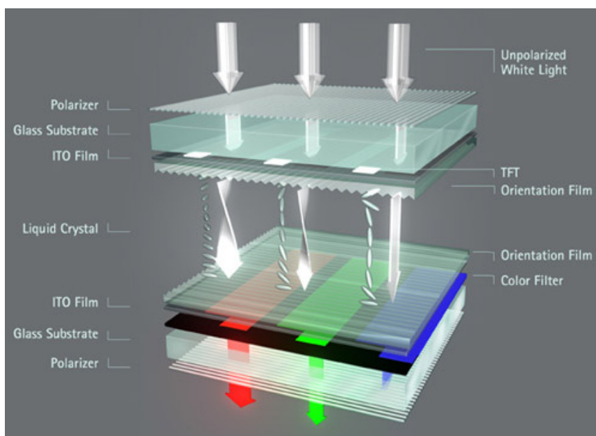
Obrázek 5: Princip činnosti barevného LCD displeje
