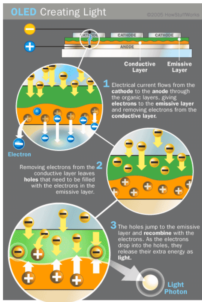
Obrázek 10: Princip činnosti organické vrstvy OLED
