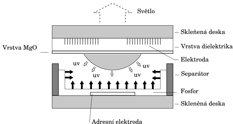
Obrázek 8: Princip činnosti jedné buňky plazma displeje
